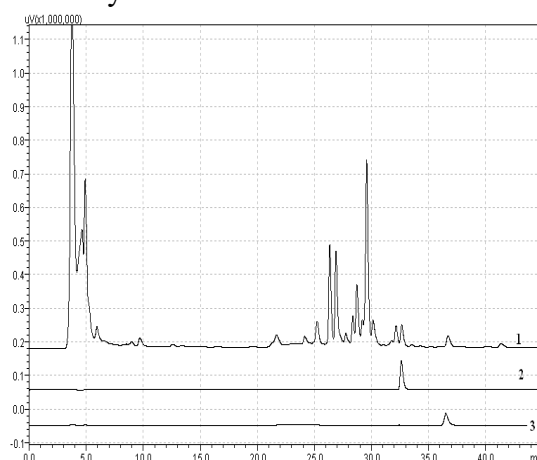
Hình 5. Hình ảnh sắc ký đồ HPLC phân tích tectoquinone và rubiadin trong mẫu ba kích (Ký hiệu: 1-SKD HPLC mẫu ba kích; 2-SKD HPLC mẫu chuẩn rubiadin; 3-SKD HPLC mẫu chuẩn tectoquinone)
