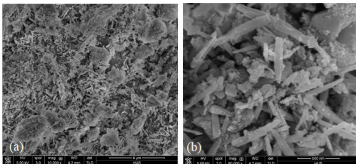
Hình 1. Ảnh SEM của vật liệu chứa \text{MnFe}_2\text{O}_4 a) Độ phóng đại 10000 lần b) 60000 lần
