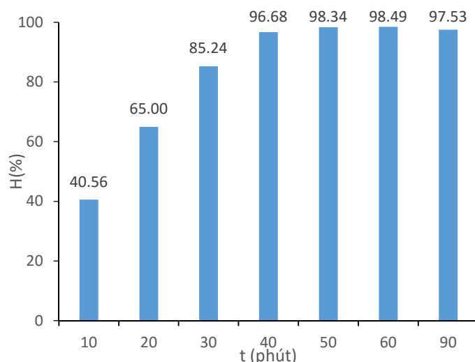
Hình 7. Khảo sát ảnh hưởng của thời gian ( pH = 2 , V = 1\text{ L} , [RY\ 160] = 50\text{ mg/L} ; hàm lượng xúc tác 0,20\text{ g/L} , [H_2O_2] = 4,9\text{ mM} , nhiệt độ 30^\circ )
