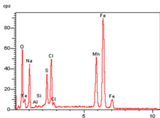
Hình 2. Phổ EDX của vật liệu chứa \text{MnFe}_2\text{O}_4
