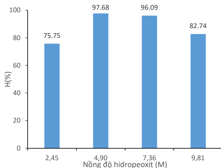
Hình 5. Khảo sát ảnh hưởng của nồng độ H_2O_2 ( pH = 2 , V = 1\text{ L} , [RY\ 160] = 50\text{ mg/L} ; hàm lượng xúc tác 0,20\text{ g/L} , nhiệt độ 30^\circ\text{C} , t = 60\text{ phút} )
