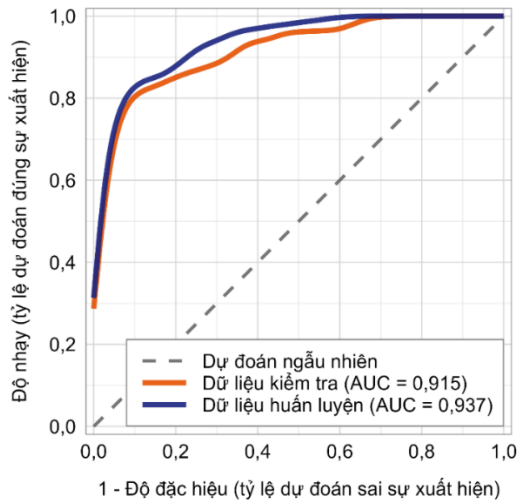
Hình 2. Đánh giá hiệu năng dự báo của thuật toán MaxEnt thông qua phân tích đường cong ROC
