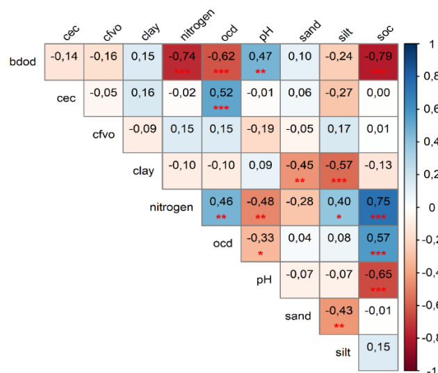
Hình 1. Tương quan giữa các đặc tính lý hóa của đất
