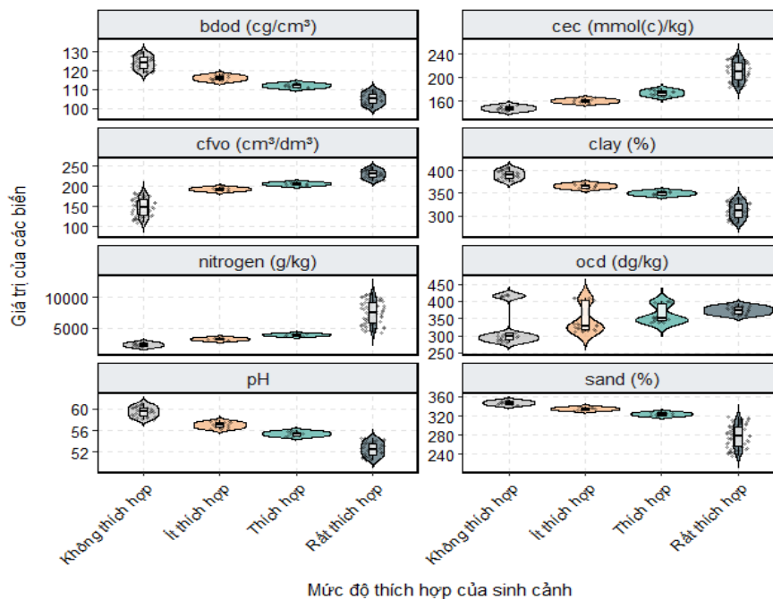
Hình 4. Phân bố mật độ của các biến thổ nhưỡng theo các mức độ thích hợp của sinh cảnh (Biểu đồ hiển thị phạm vi biến động dữ liệu qua 3 lớp. (1) Các chấm tròn nhỏ đại diện cho từng điểm dữ liệu, thể hiện phạm vi biến động tuyệt đối từ giá trị nhỏ nhất đến lớn nhất. (2) Hình dáng violin minh họa mật độ phân bố; phần phình to chỉ định khu vực tập trung nhiều dữ liệu nhất. (3) Hộp chữ nhật (boxplot) thể hiện khoảng phân bố của 50% dữ liệu cốt lõi, với đường gạch ngang đậm là giá trị trung vị (median). Hai thanh râu (whiskers) kéo dài từ hộp đại diện cho giới hạn dữ liệu chuẩn)
