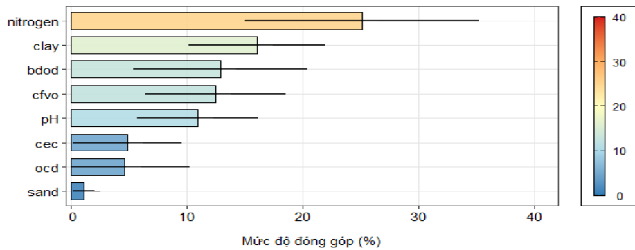
Hình 3. Mức độ đóng góp của các đặc tính lý hóa đất vào mô hình dự báo MaxEnt (Độ dài của các cột thể hiện giá trị đóng góp trung bình của từng biến; màu sắc cột minh họa trực quan mức độ quan trọng từ cao xuống thấp. Các thanh sai số màu đen thể hiện khoảng biến thiên của dữ liệu qua các lần hoán vị)
