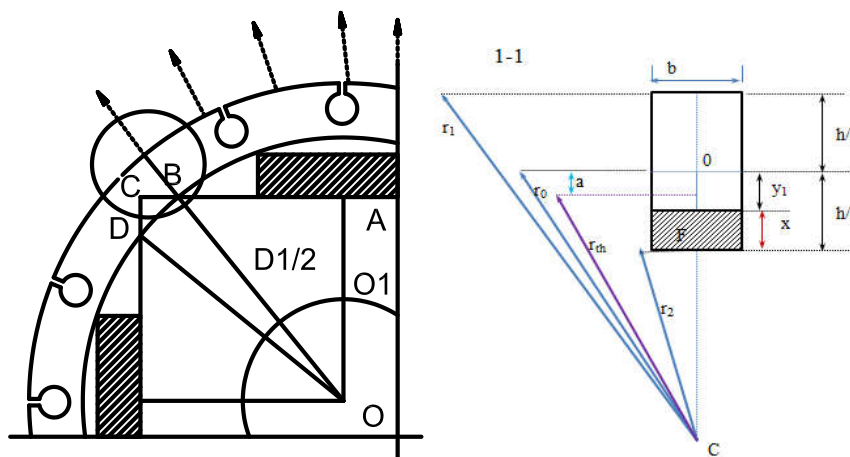
Hình 8. Mặt cắt xác định các kích thước để tính ứng suất
